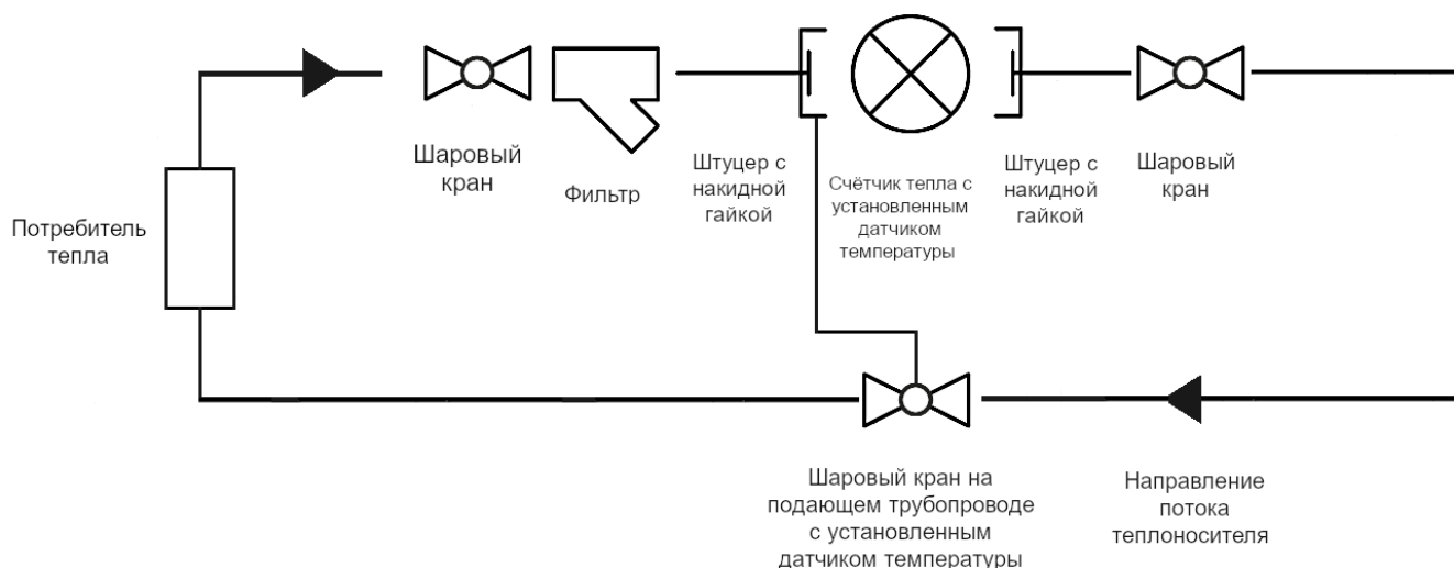
Рис 2 (Б) – Установка счётчика на обратный трубопровод
